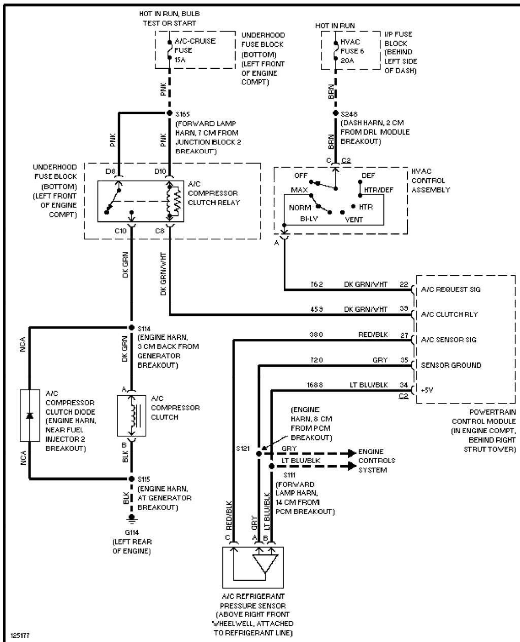
3.8L VIN K, Compressor Circuit
